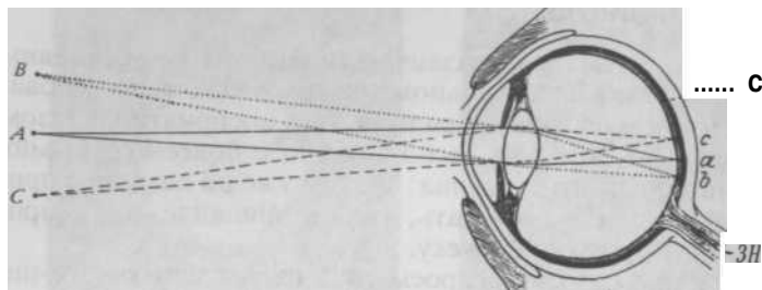
Рис. 54. Глаз человека. С — сетчатка; ЗН — зрительный нерв. (Объяснение в тексте.)
