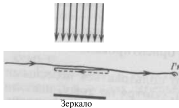
Рис. 73. Опыт с зеркалом доказывает, что муравьи ориентируются по солнцу. Пунктирная линия — путь муравья, когда он видит отражение солнца в зеркале. Гн — гнездо. (По Санчи.)
