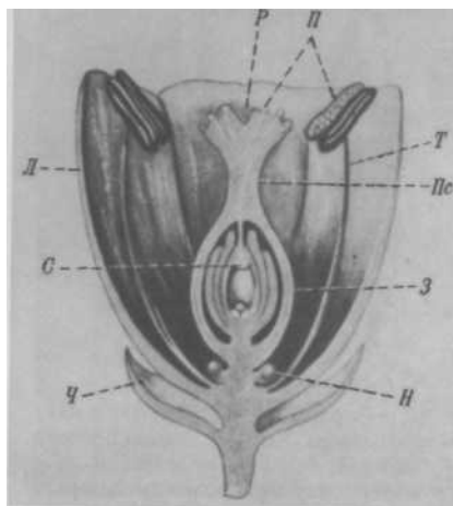
Рис. 19. Цветок, разрезанный вдоль через центр. С — семяпочка; З — завязь; Пс — пестик; Р — рыльце; П — пыльник; Т — тычинка с пыльниками; Л — лепестки; Ч — чашелистики; Н — нектар.
