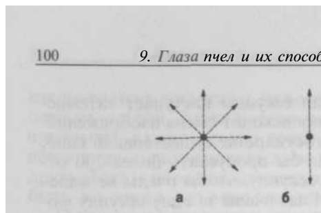
Рис. 60. Схема, поясняющая отличие обычного света (а) от поляризованного (о) (см. текст).
