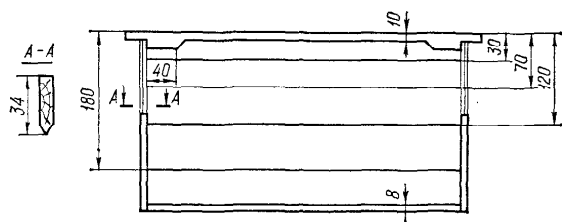
Рис. 5. Рамка (размеры — в мм)
