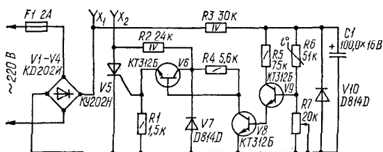
Рис. 3. Принципиальная схема терморегулятора
