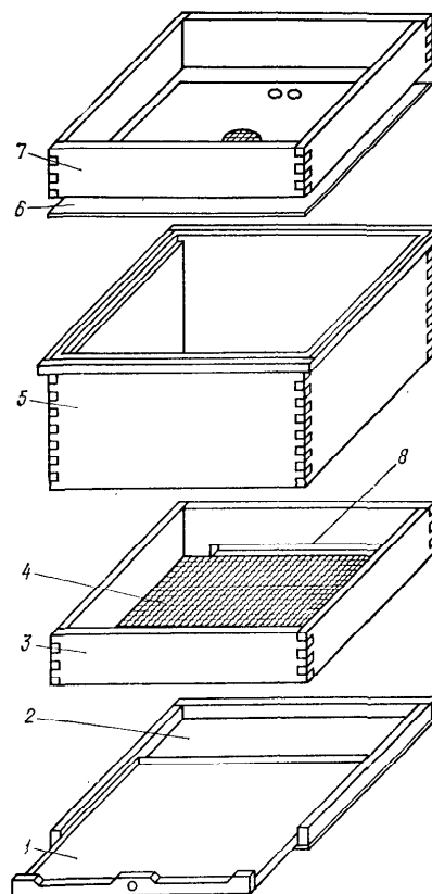
Рис. 4. Состав улья: 1 — поддон; 2 — дно; 3 — подставка; 4 — сетка; 5 — корпус; 6 — потолок; 7 — подкрышник; 8 — леток
