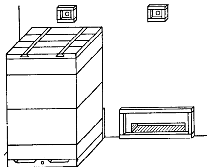
Рис. 6. Улей в павильоне и оформление летка в стене павильона
